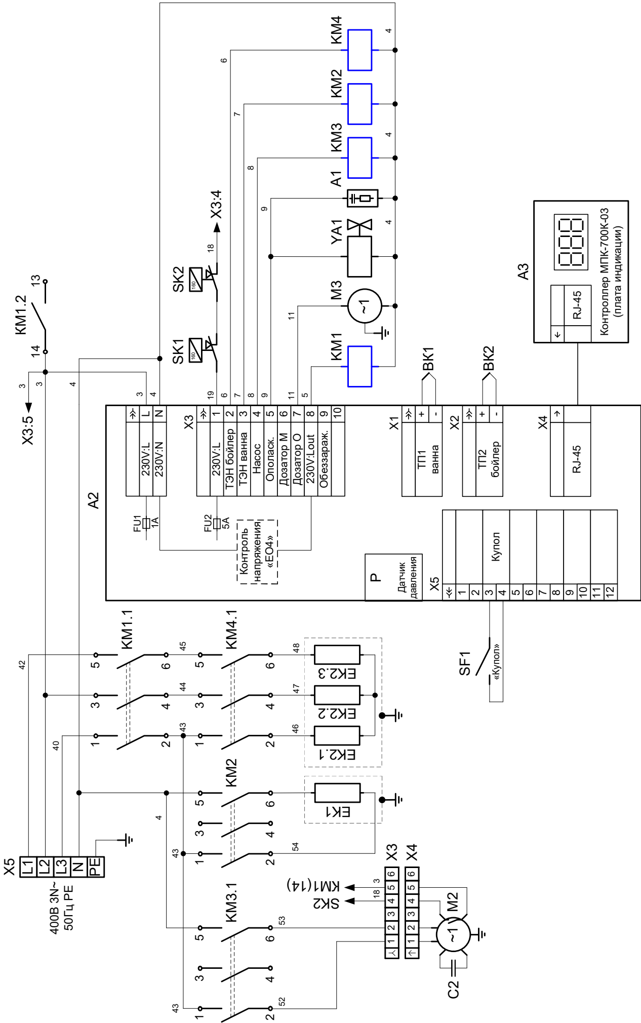
10 СХЕМА ЭЛЕКТРИЧЕСКАЯ ПРИНЦИПИАЛЬНАЯ МАШИН МПК-700К-01, МПК-700К-03
