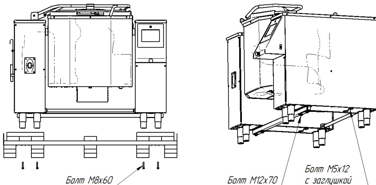
Рис. 4 Распаковка и установка котла
