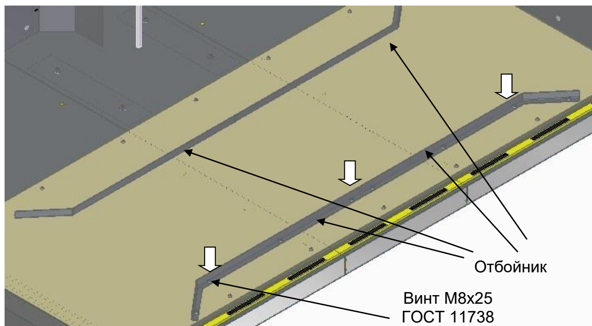
Рис. 26 Установка отбойника
