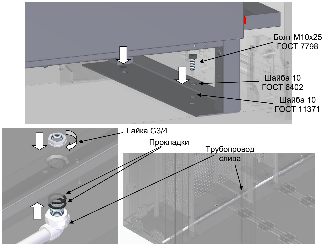
Рис. 17 Монтаж воздухоохладителей и системы слива
