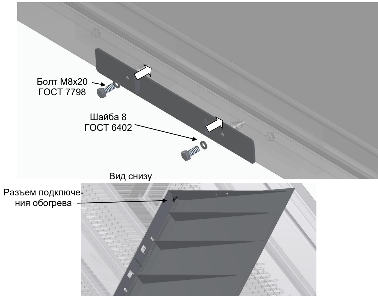
Рис. 25 Установка пандуса
